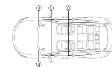
⑥ 9cm スコーカー ⑦ 18cm ドアスピーカー ⑧ 16cm ドアスピーカー ⑨ 20cm サブウーハー 6スピーカーレイアウト
