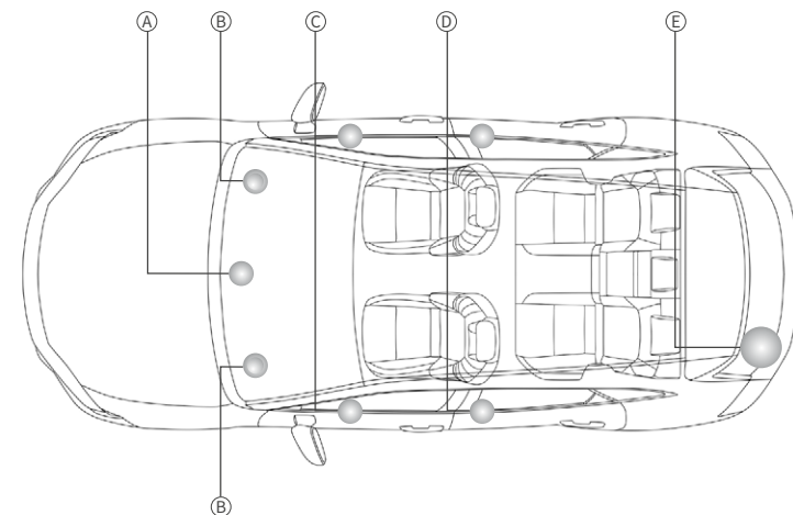
(A) 9cmスコーカー (C) 18cmダブスピーカー (B) コアキシャル9cmスコーカー (D) 16cmダブスピーカー +2.5cmツイーター (E) 20cmサブウーハー
