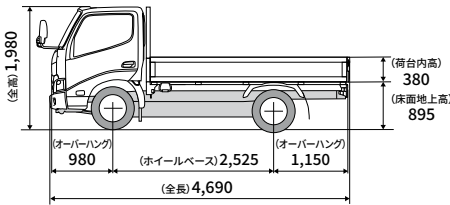
■寸法図(単位:mm) 2SG-XKC605-TQVMY 車型番号 89
