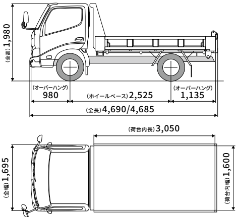
■ 寸法図 (単位:mm) 2WG-XZU676C-TWMMJ 車型番号 4
