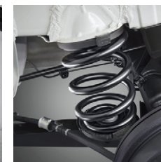
トレーリングリンク式 リアコイルサスペンション
