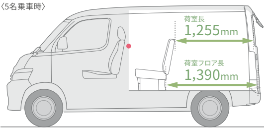
荷室長・荷室フロア長
